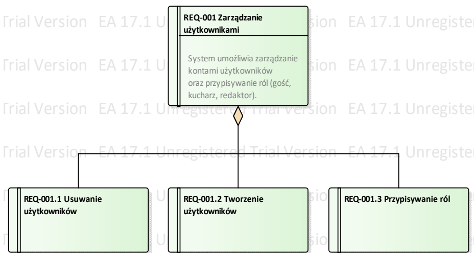
Figure 4: Diagram hierarchiczny zarządzania użytkownikami
