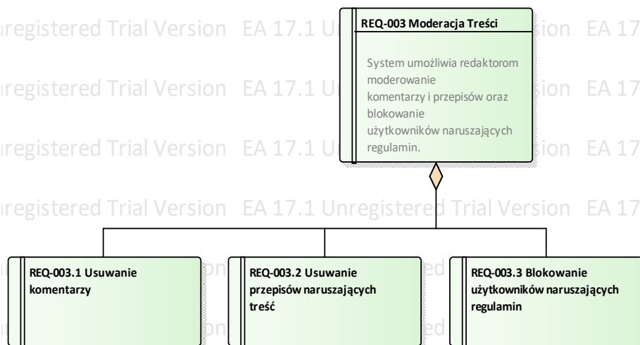
Figure 2: Diagram hierarchiczny moderacji treści
